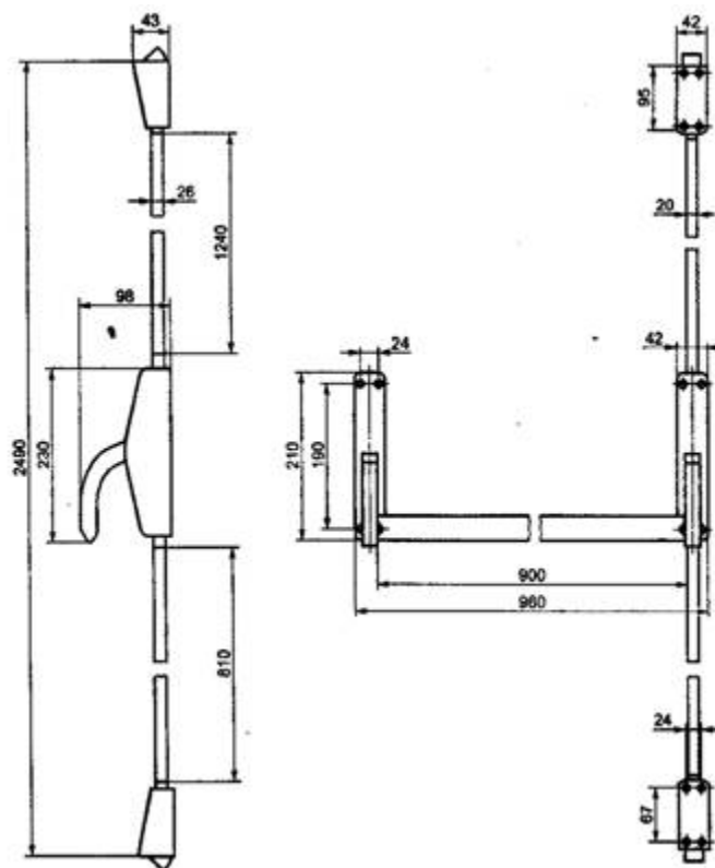
Рисунок А.3 – Пример устройства «Антипаника», управляемого штангой с запириением дверей эвакуационных выходов в трех точках.
